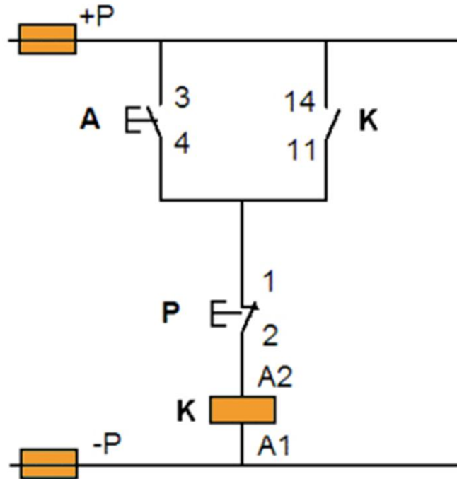
Esquema de Principio
