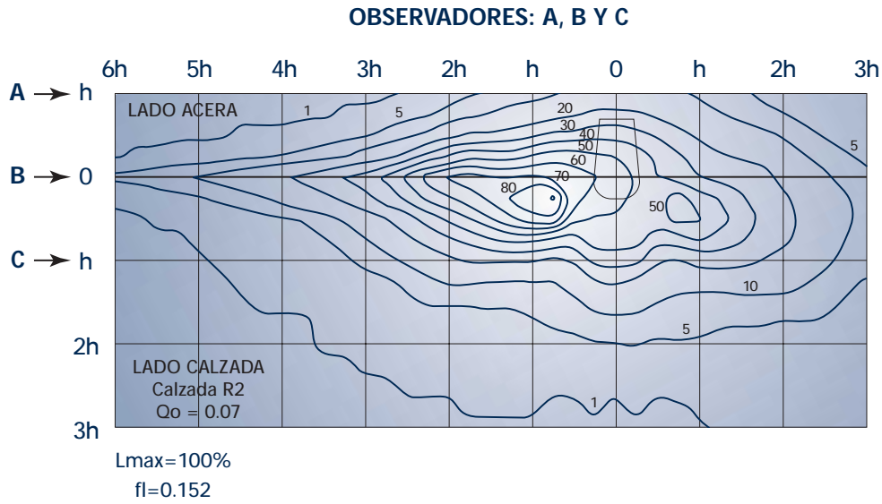
Figura 14. Curvas isoluminancias.
