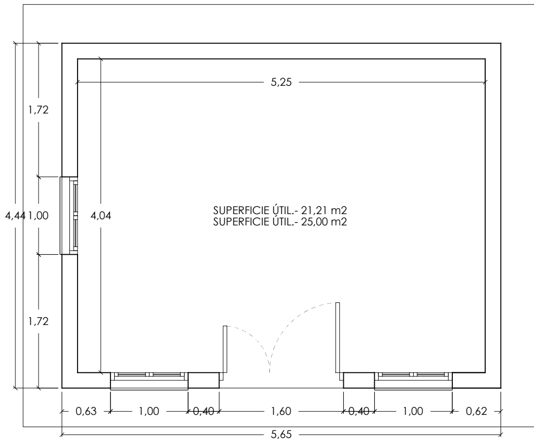
PLANTA GENERAL
