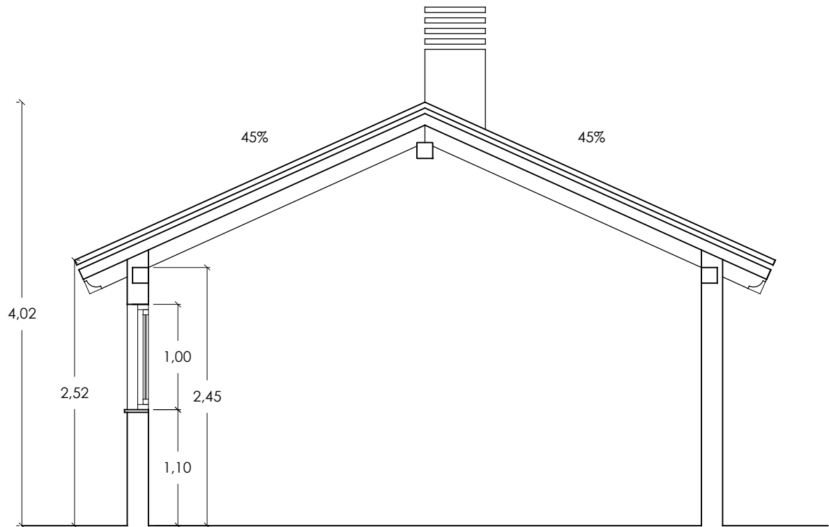
SECCIÓN GENERAL
