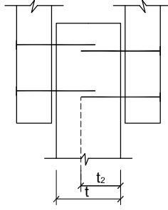
Figura 8.6 Solape de clavos.
