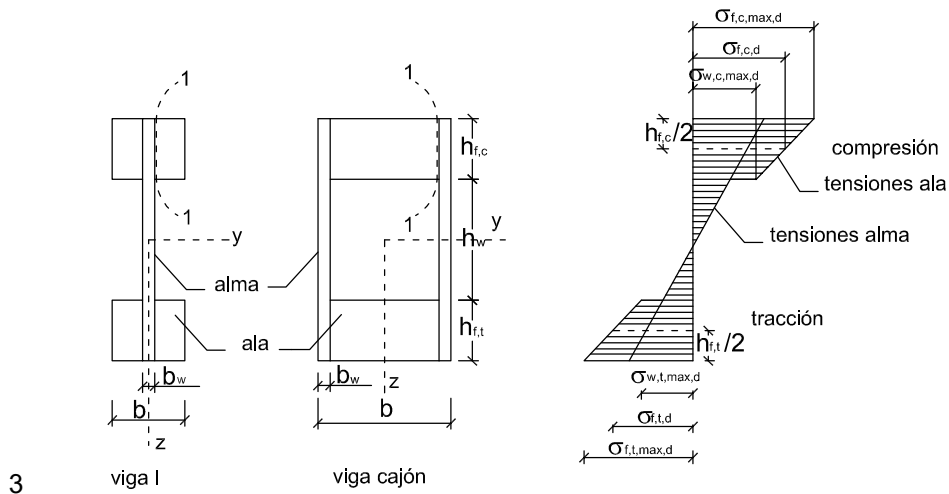
Figura 10.1 Vigas en I ó doble T y cajón de alma delgada formada por tableros
