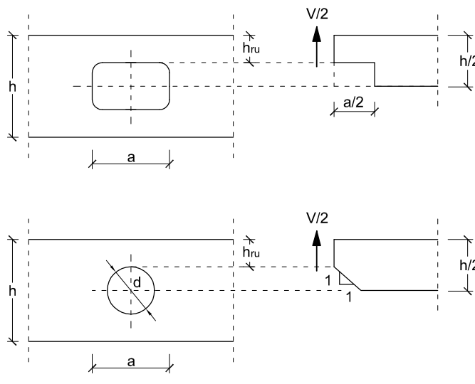
Figura 6.18 Las vigas con agujeros situados en el centro de la viga se comprobarán a cortante considerando un efecto equivalente como si se tratara de una entalladura en la viga. A la izquierda se representan los agujeros y a la derecha la entalladura equivalente.
