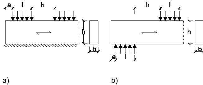
Figura 6.2 Longitud eficaz a compresión perpendicular a la fibra. a) durmiente (apoyo en continuo) y b) apoyo aislado.
