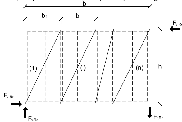
Figura 10.7 Muro diafragma
